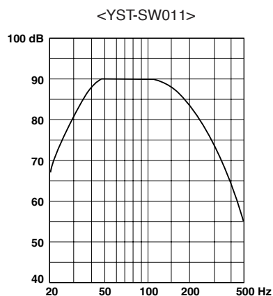
Graphique de réponse en fréquence*
